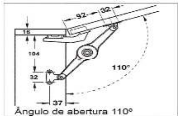
Empurrar o botão para permitir que os braços girem no sentido das setas e alterar de porta elevatória para abatível
