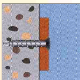
4 - Trabalho terminado
