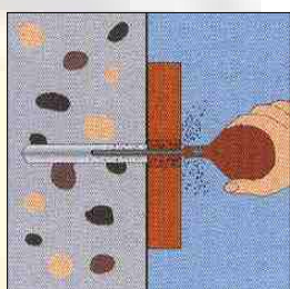
2 - Limpar o furo
